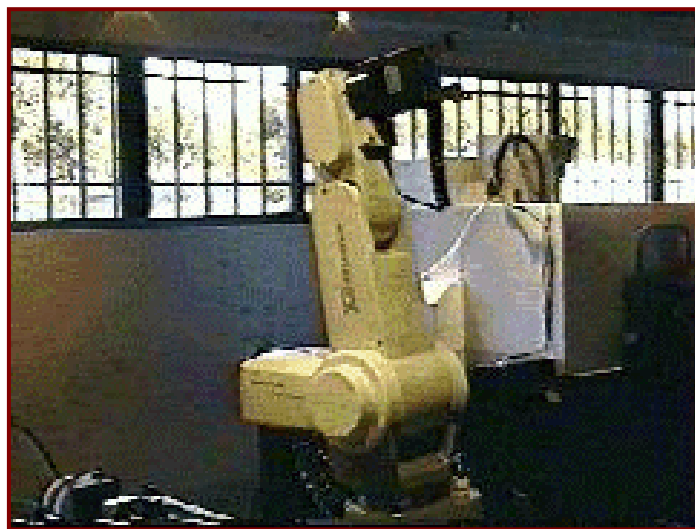
Figura 1. El robot Mitsubishi es de tipo brazo articulado y tiene 5 articulaciones. El principal uso de este robot es para ensamble y carga/descarga de piezas a la estación de medición.
