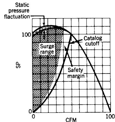
Fig 14-27. Fan surge
