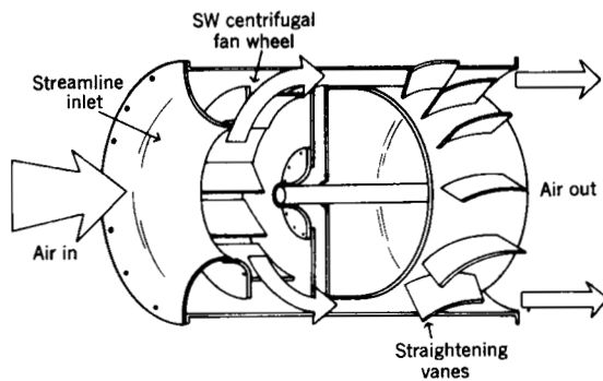
Fig 14-37. Tubular centrifugal fan
